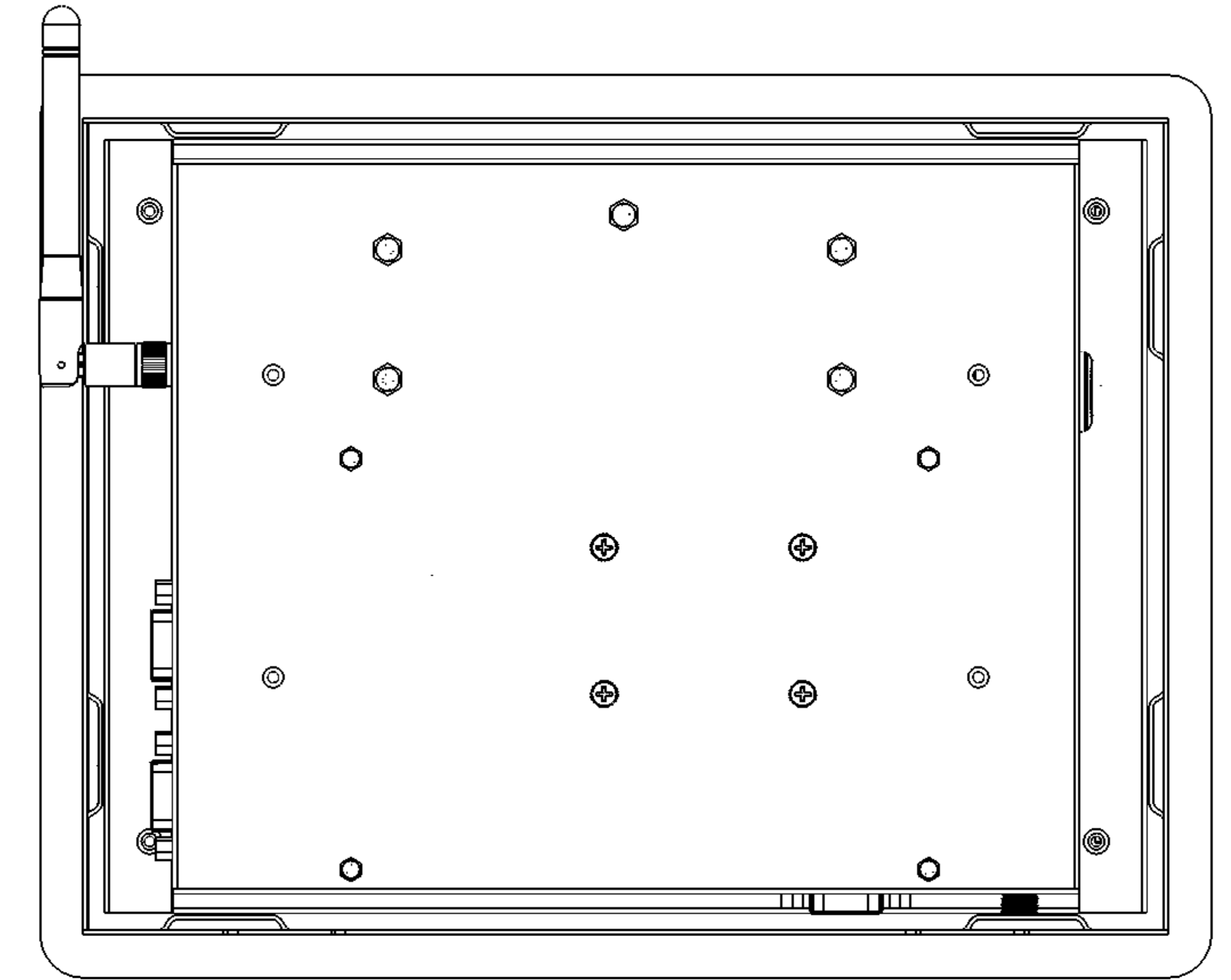
视图 A
