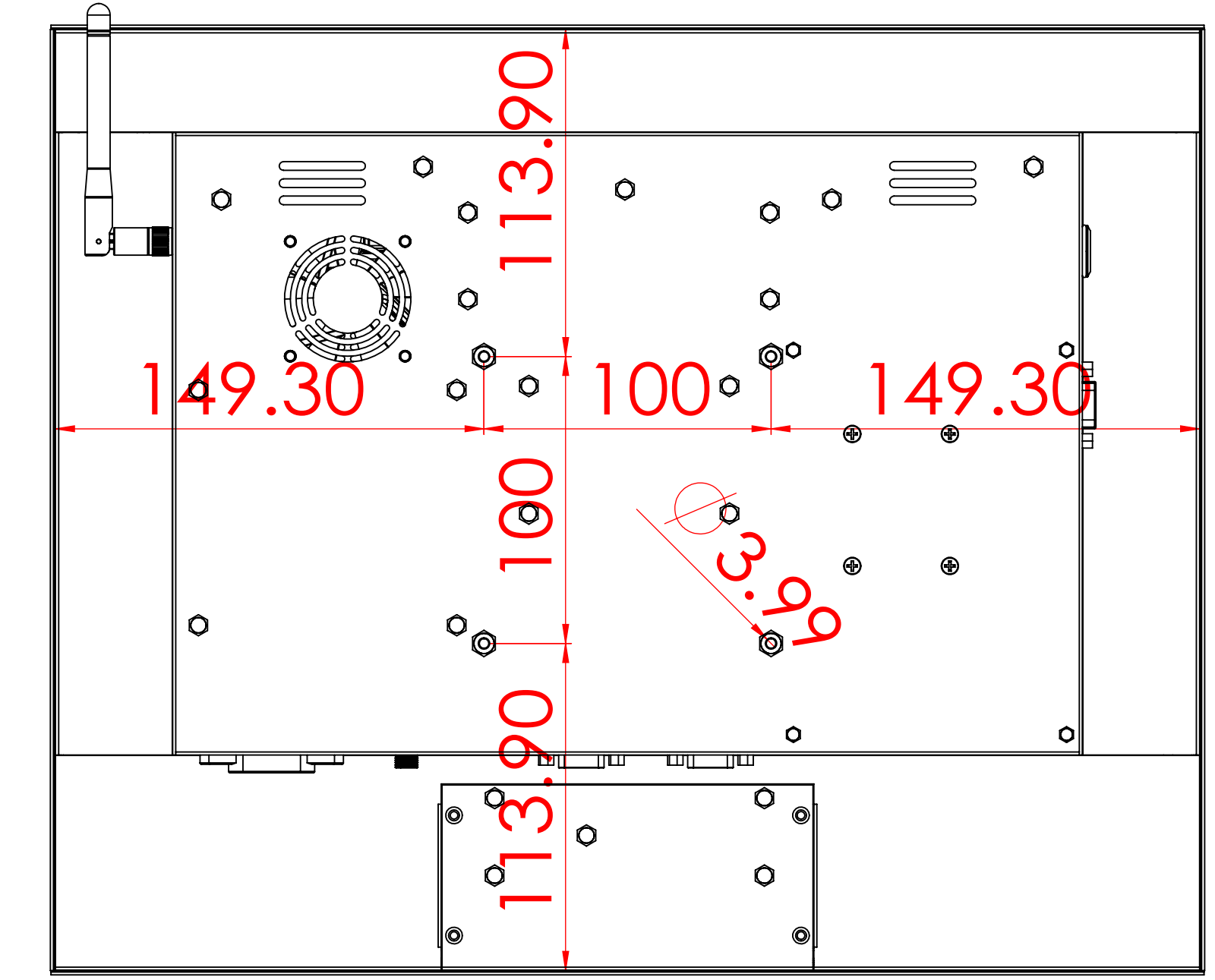
视图 A
