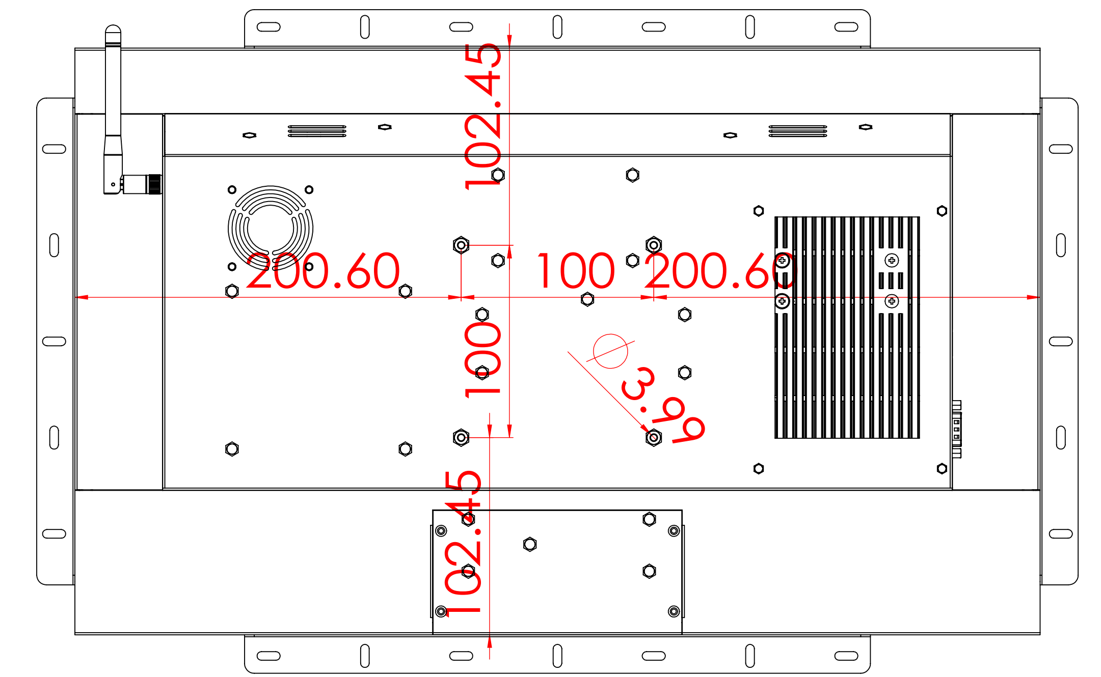
视图 A
