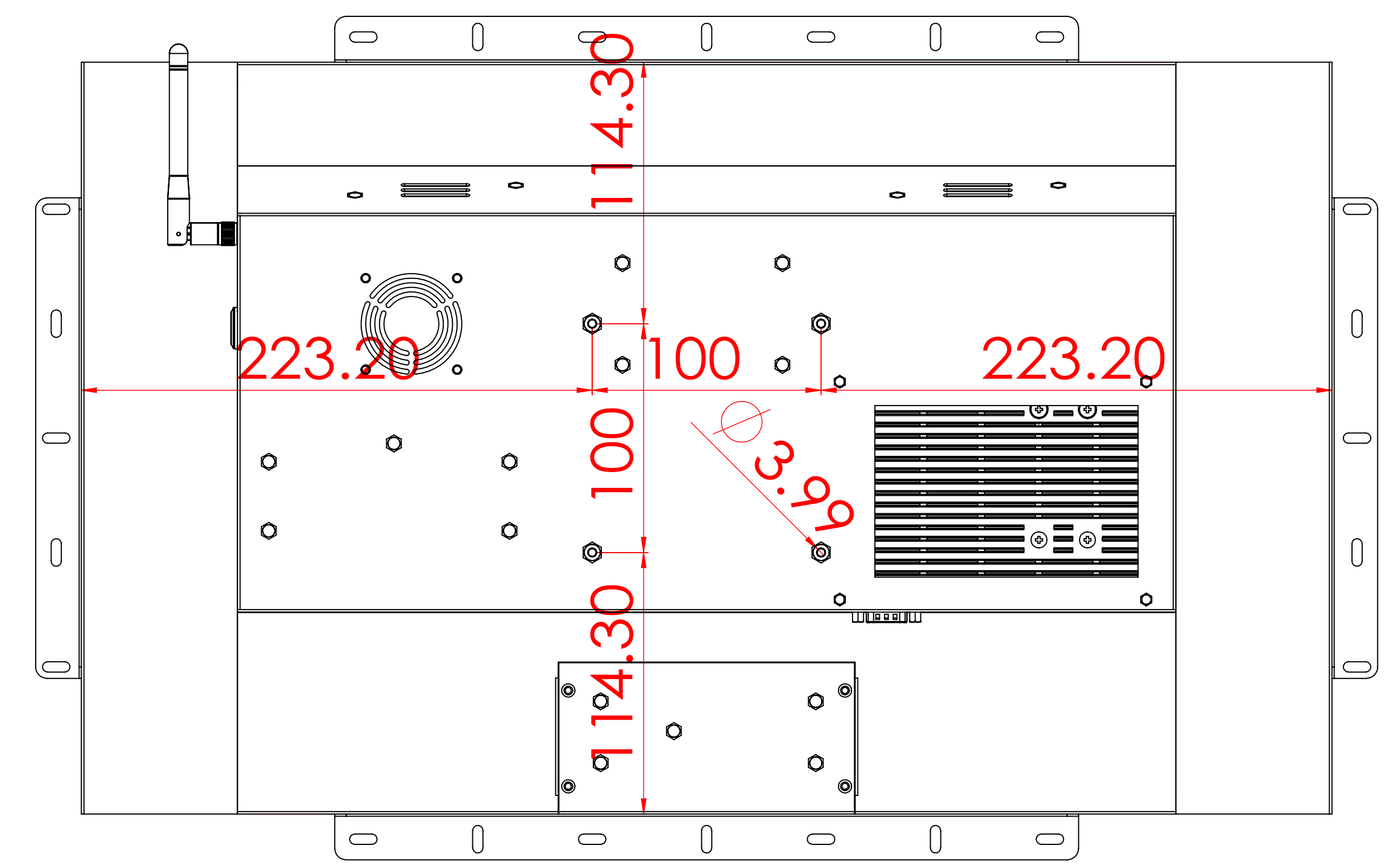
視圖 A
