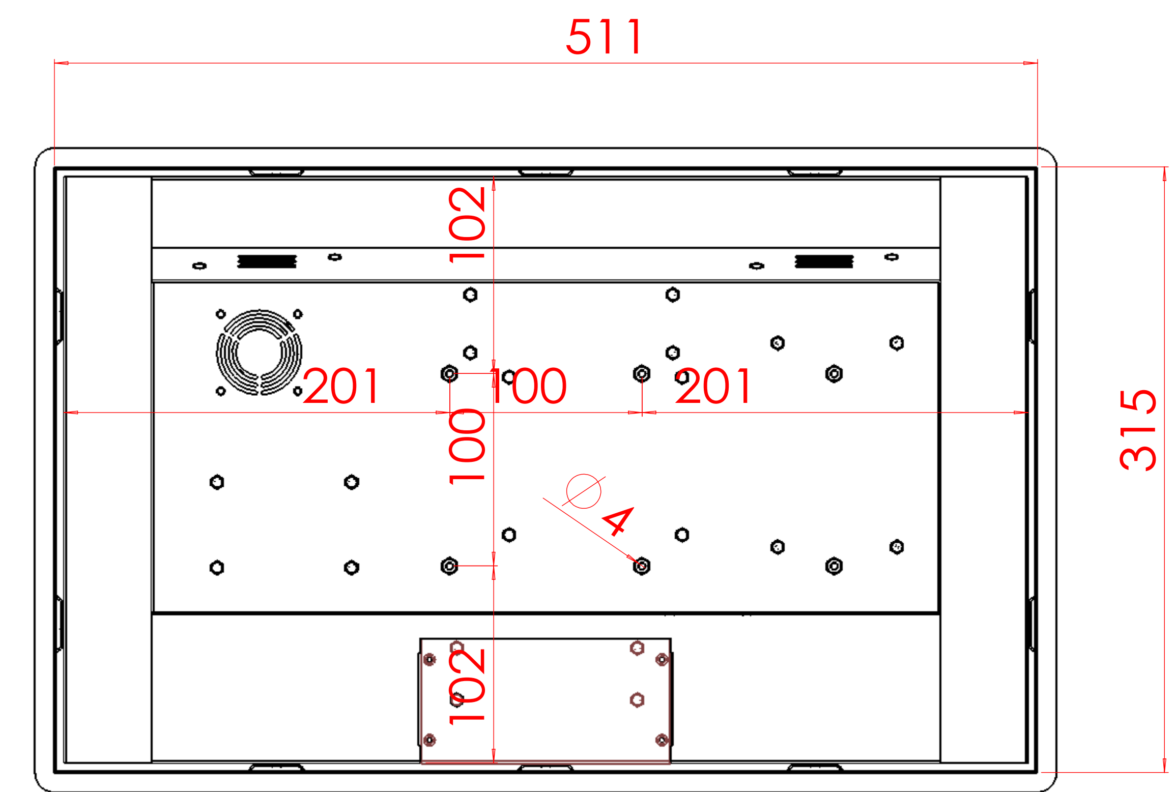
視圖 A
