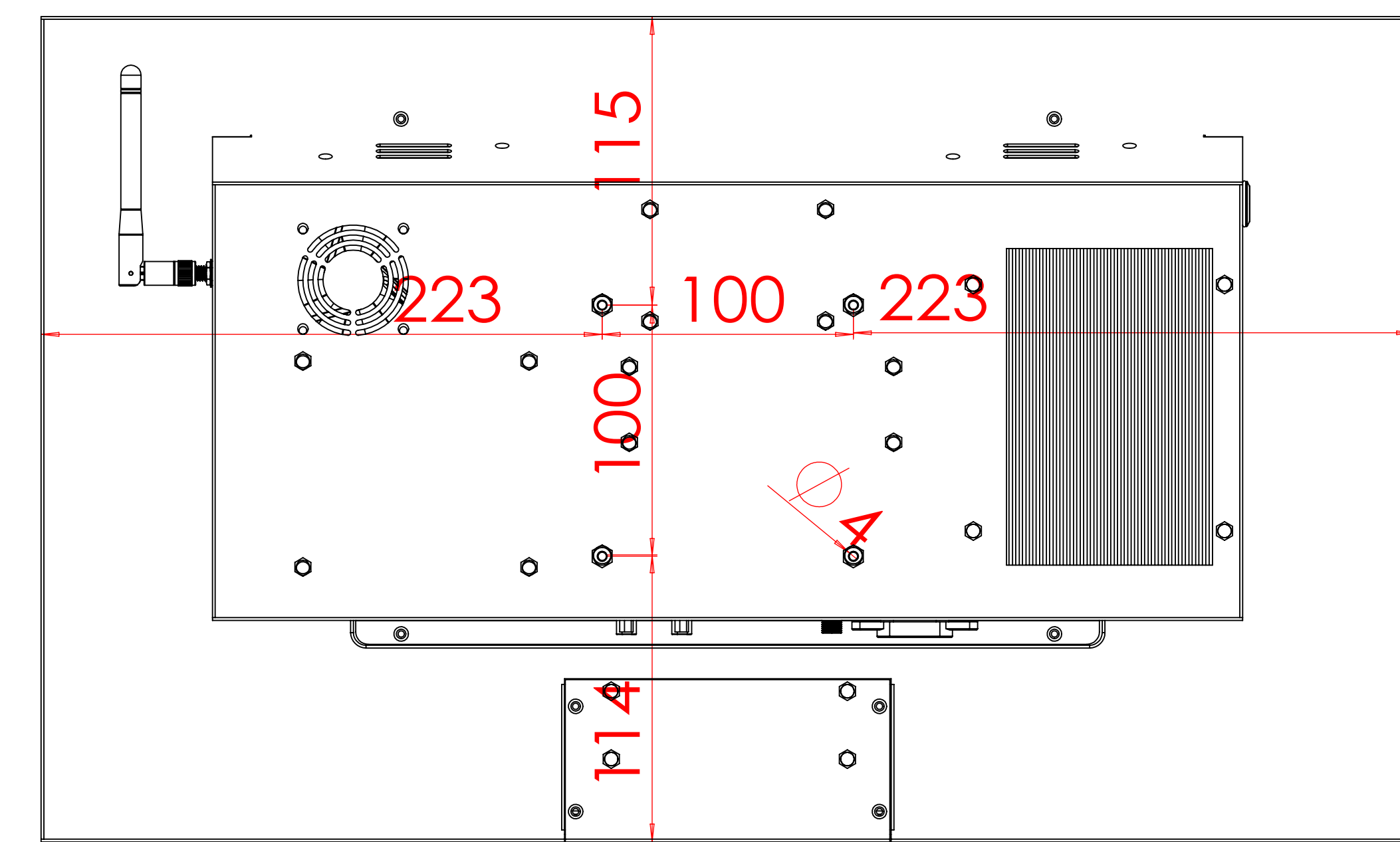
視圖 A
